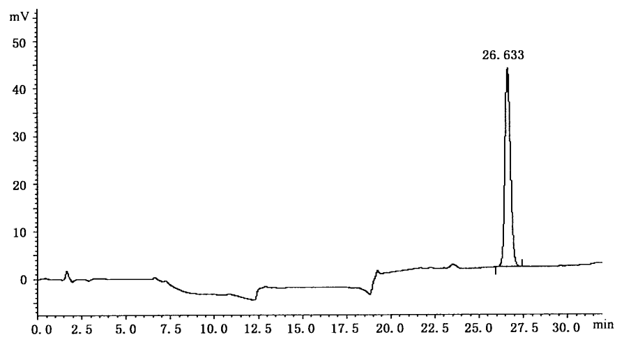
图 A.1 刀豆氨酸标准色谱图(20 µg/mL)
