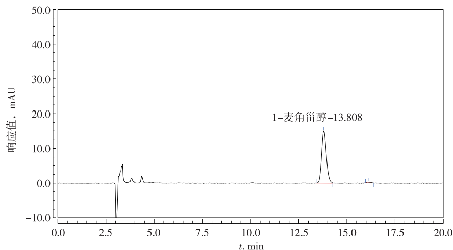
图 A.1 麦角甾醇标准溶液 (10 μg/mL) 高效液相色谱图
